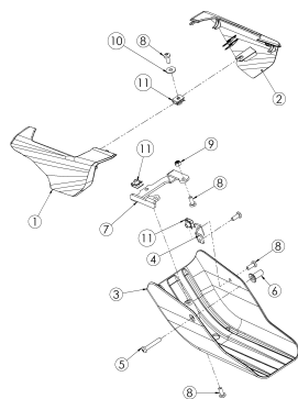
Lámina 13 - PLASTICOS (Subchasis & Protector inferior)
