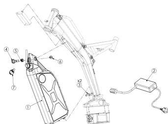
Lámina 11 - BATERIA DE POTENCIA
