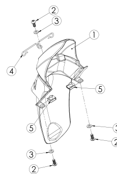
Lámina 14 - PLASTICOS (Guardabarros trasero)
