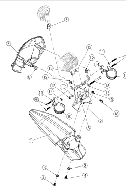
Lámina 12 - PLASTICOS (Portafaro & Guardabarros delantero)
