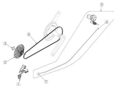
Lámina 10 - TRANSMISION
