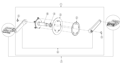
Lámina 15 - PEDALIER
